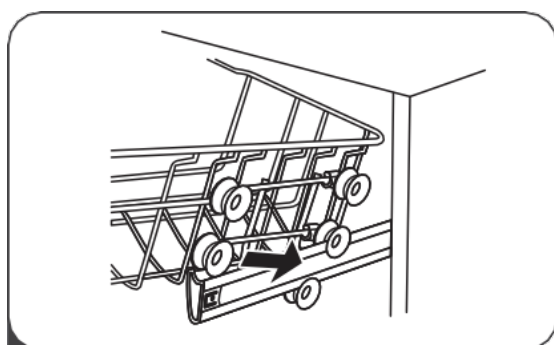
3 Sätt tillbaka den övre korgen på övre eller undre valsarna.
